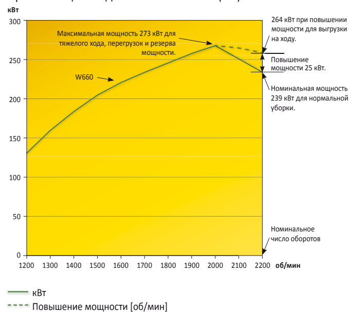
Кривая мощности двигателя PowerTech (9 л)
